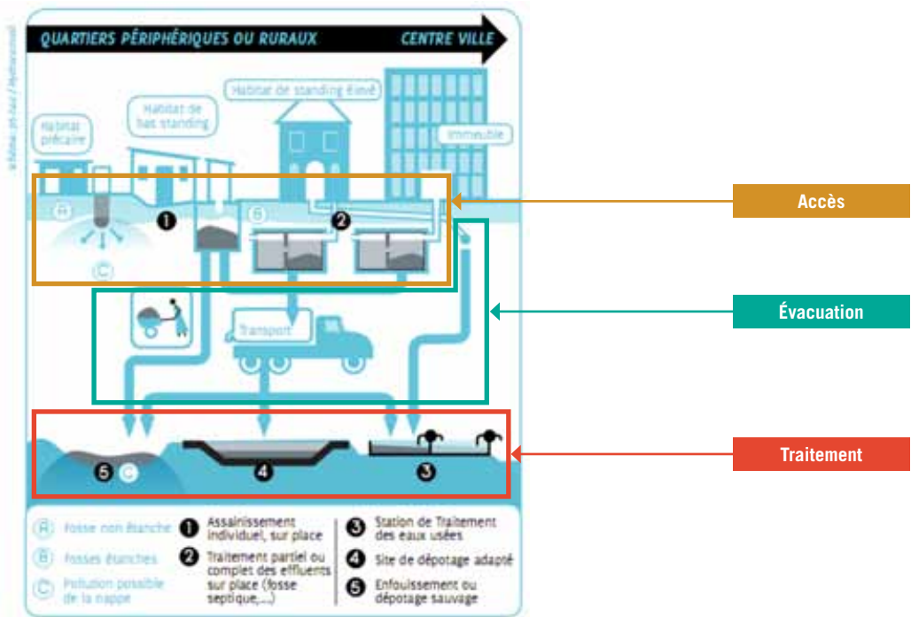
FIGURE N° 4 Les trois maillons successifs des filières d'assainissement Source : pS-Eau
