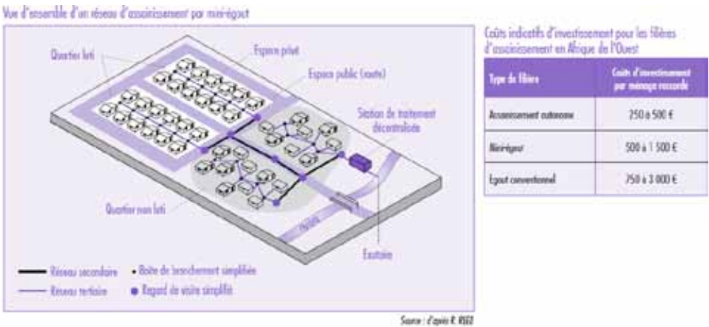
FIGURE N° 9 Schématisation du tracé d'un réseau de mini-égouts et analyse comparée des coûts d'investissement standards en Afrique de l'Ouest Source : L'Équipe R. R&D, 2014, p. 9 et 26
