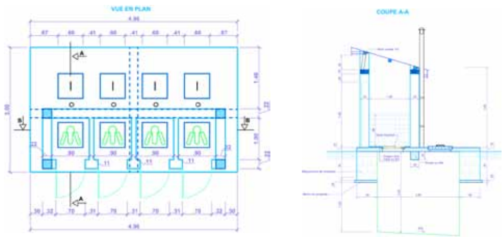
FIGURE N° 5 Bloc sanitaire d'une école à Ambohibary (Madagascar) Source : Gret
