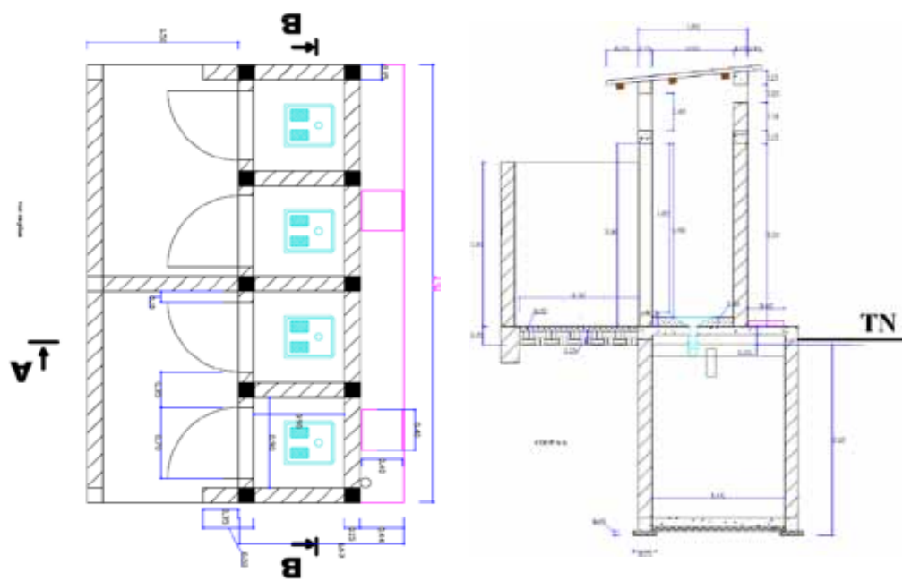
FIGURE N° 4 Bloc sanitaire d'une école à Rosso (Mauritanie) Source : Gret
