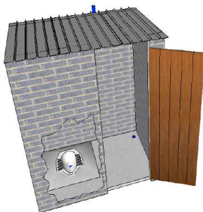
Modèle d'installation domiciliaire « latrine+douche »
