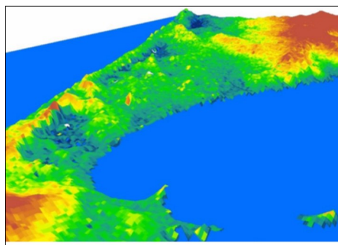
Vue en 3D des bassins versants dans les départements de Pikine et Guédiawaye (sources: Gret, DGPRE)
